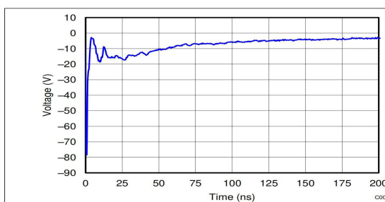
图 5-7. -8-kV IEC Waveform
