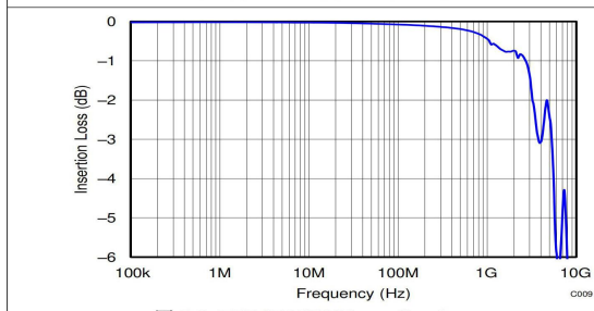
图 5-9. TPD4E05U06 Insertion Loss
