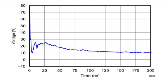
图 5-6. 8-kV IEC Waveform
