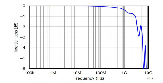
图 5-10. TPD6E05U06 Insertion Loss
