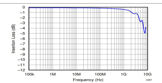
图 5-8. TPD1E05U06 Insertion Loss
