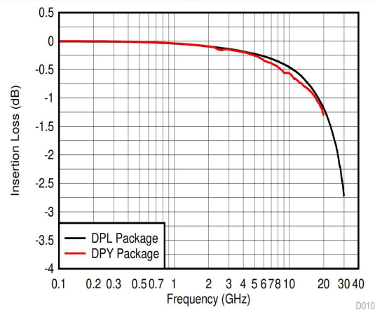
图 5-11. 插入损耗
