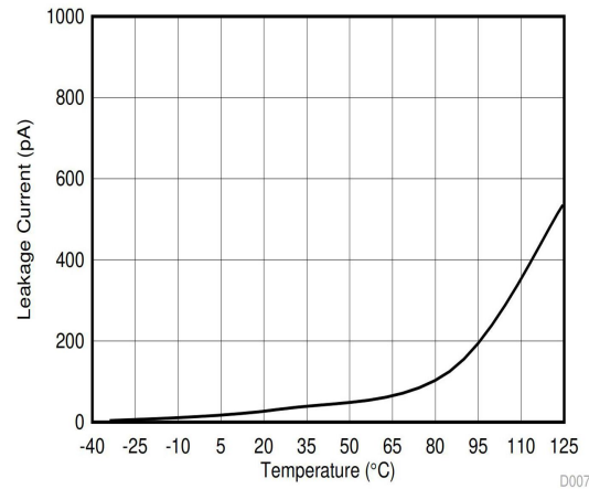
图 5-8. 漏电流与温度间的关系
