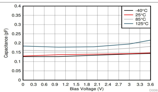
图 5-6. 电容与偏置电压间的关系 (DPL 封装)
