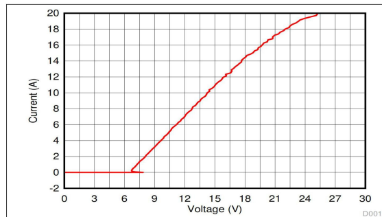
图 5-1. 正 TLP 曲线
