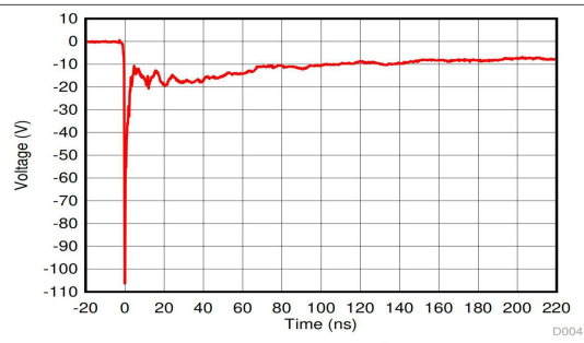
图 5-4. -8kV IEC 波形
