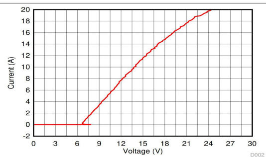
图 5-2. 负 TLP 曲线
