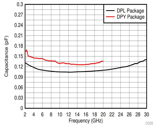
图 5-10. 电容与频率间的关系
