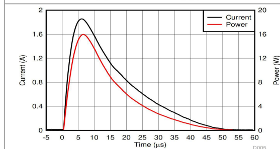
图 5-5. 浪涌曲线 ( t_p = 8/20\mu s ), IO 引脚至 GND
