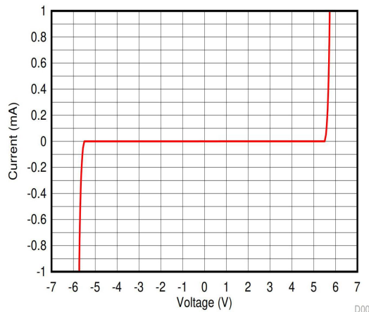
图 5-9. 直流电压扫描 I-V 曲线
