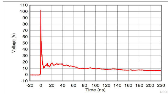
图 5-3. 8kV IEC 波形
