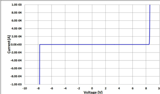
图 5-5. IV Curve
