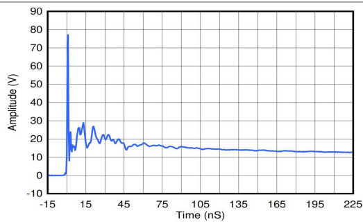
图 6-1. ESD Clamp Voltage +8 kV Contact ESD
