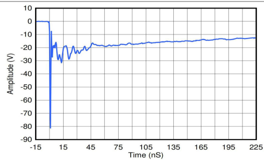
图 6-2. ESD Clamp Voltage -8 kV Contact ESD
