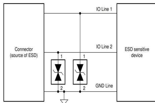
应用原理图
