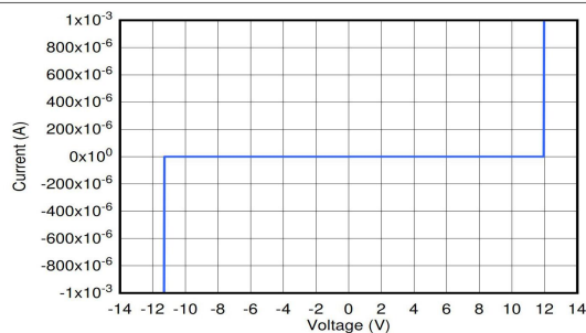
图 6-5. IV Curve
